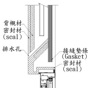
圖 R10.10 開口板片上方之別水接縫圖例 (立剖面)
