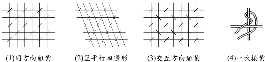
圖 R5.2 鋼筋綁紮之方向 [5.1]
